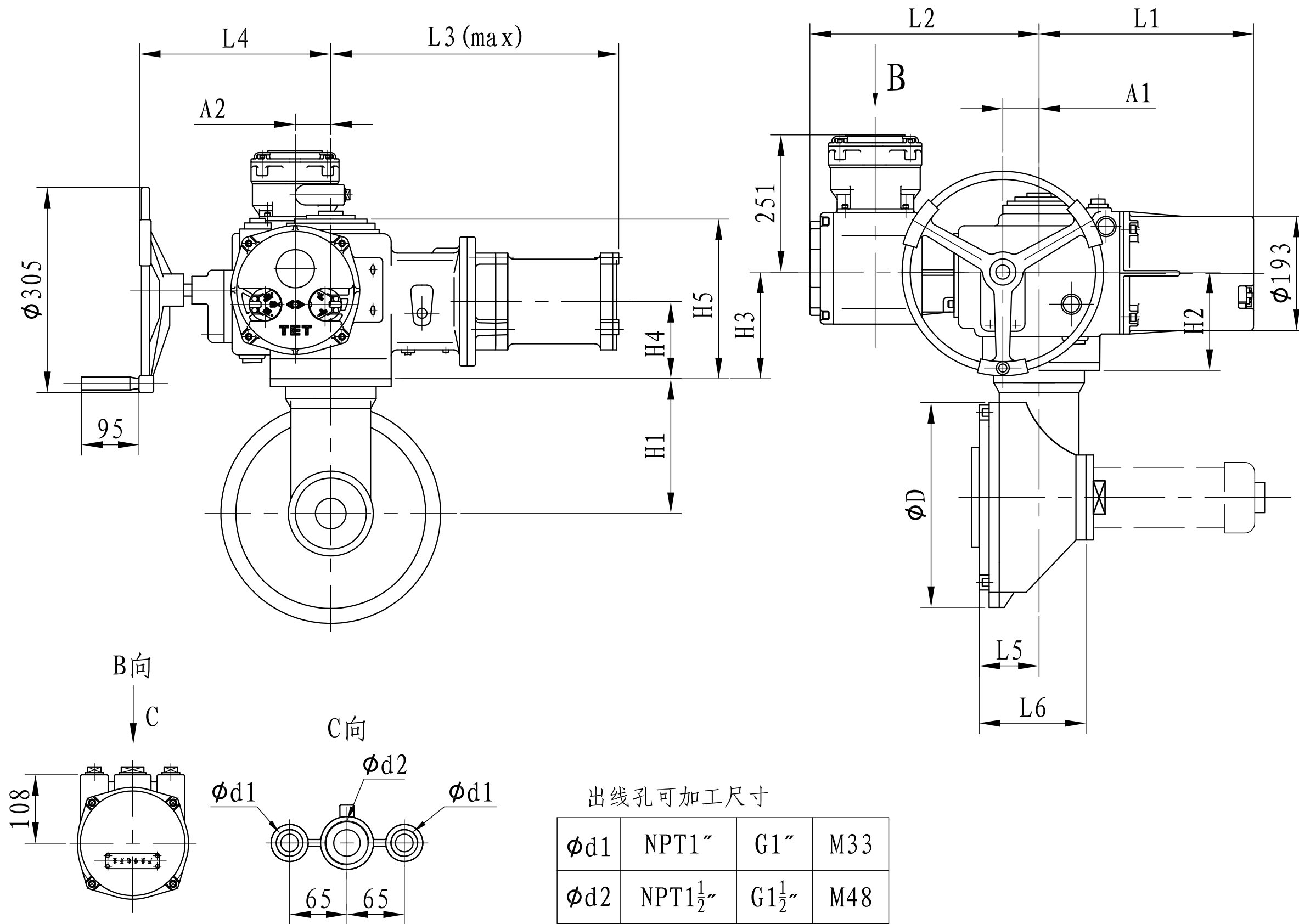
IMT-00/BA、IMT0-BA外形尺寸图
